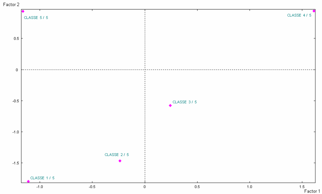
Gráfico 18. Representación de las clases obtenidas
