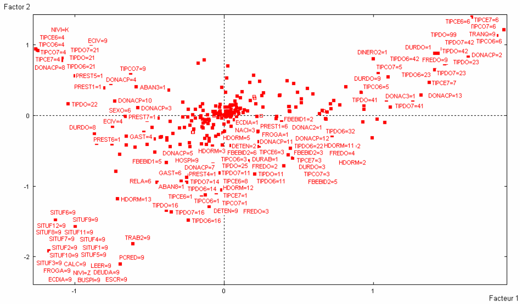
Gráfico 15. Representación del plano factorial
